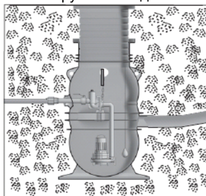
Рис. 9. Трубные соединения.
